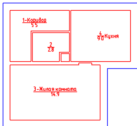
План 1 этажа
