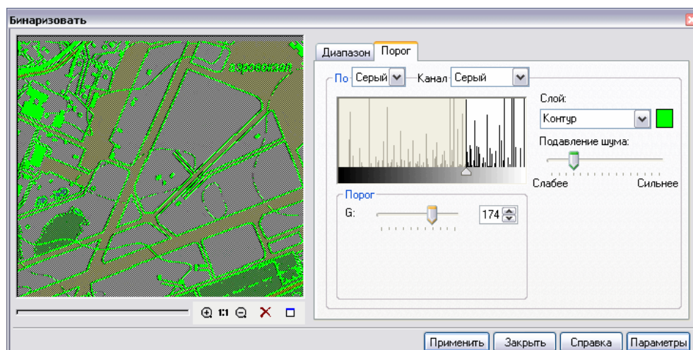
Пороговая бинаризация
